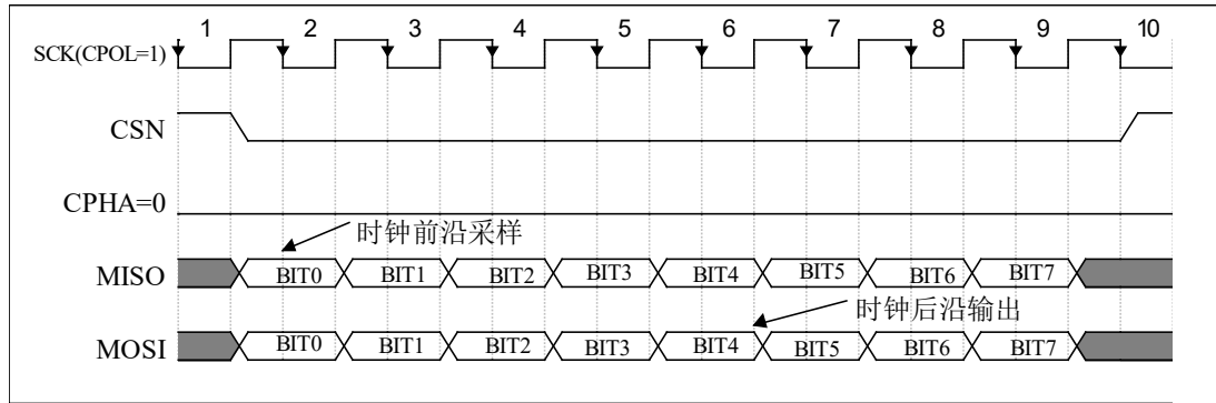
图 13-3 spi 模式 2 时序图
