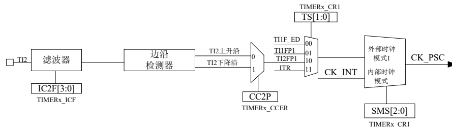
图 9-19 TI2 外部时钟连接例子
