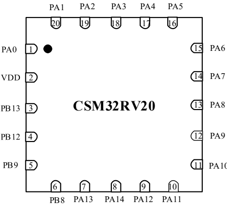
图 1-4 管脚信息图（3x3 mm QFN20）
