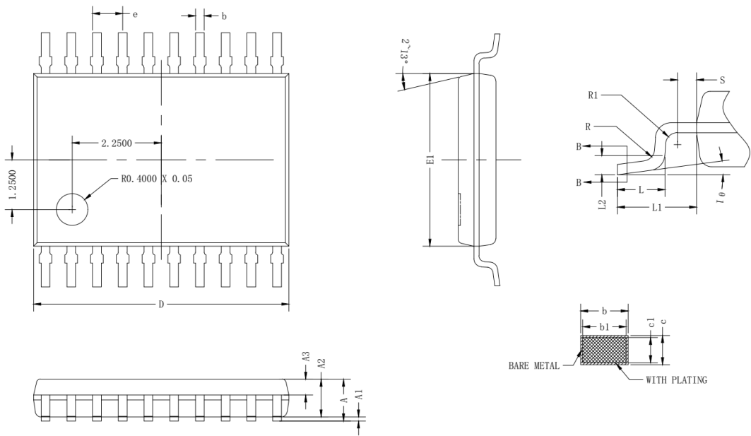
图 25-2 TSSOP20 封装
