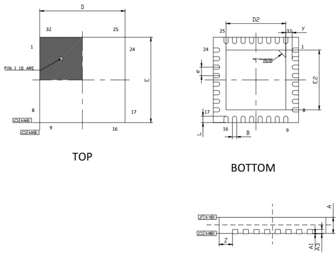
图 25-1 QFN32 封装
